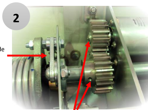
Fixations des pignons « moteur » (1 vis axiale) et « arbre » (2 vis radiales à 120°)
