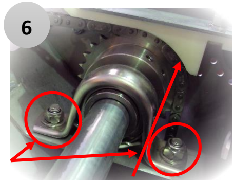
Fixation des pignons (2x) « chaîne » (2 vis radiales à 120°)
