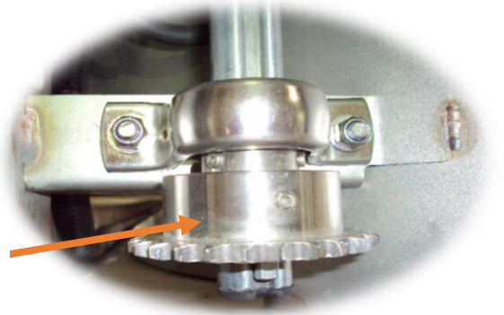
Pignon d'entraînement du tablier (par chaînes)
